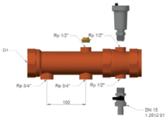
Рис. 5 - Четное кол-во отводов
