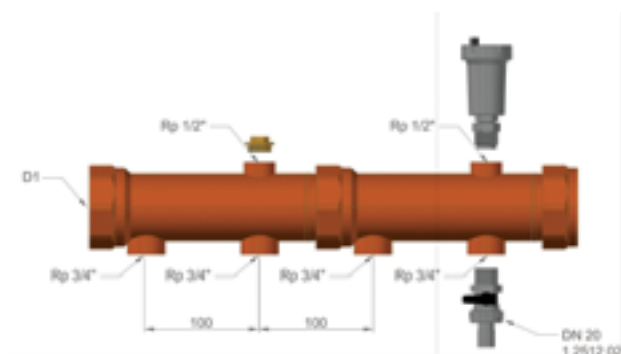
Рис. 4 - Нечетное кол-во отводов
