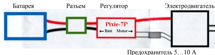
Схема подключения регулятора
