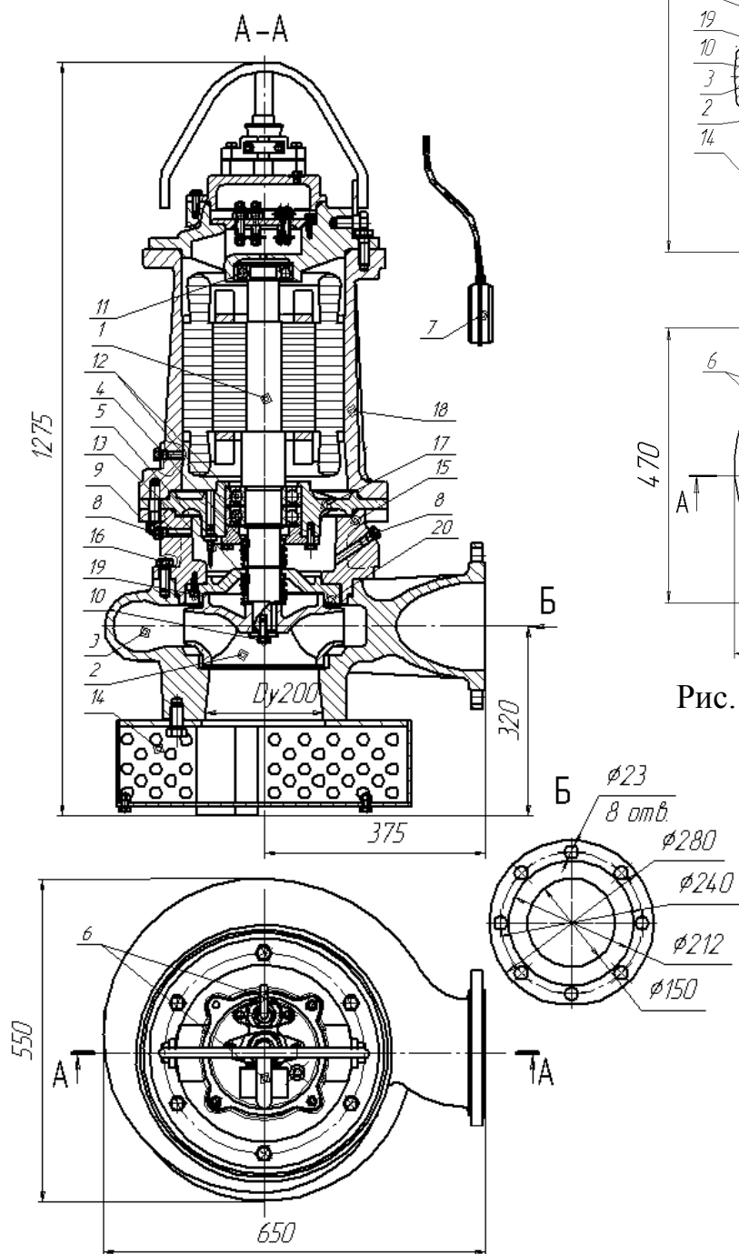
Рис. 17 Общий вид, габаритные и присоединительные размеры электронасоса "Иртыш" ПД 150/250 – 18,5/4.
