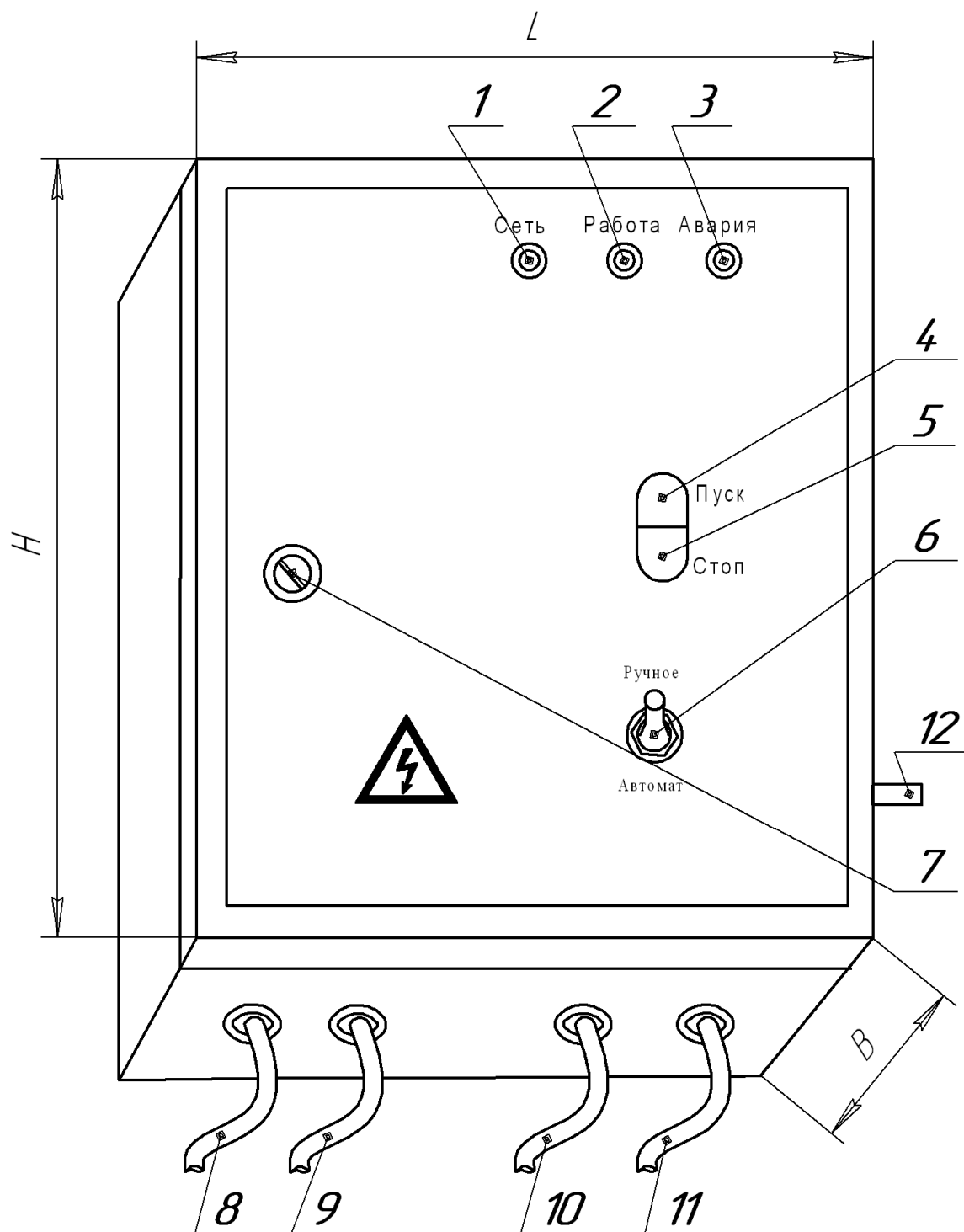
Рис. 29 Общий вид щита управления электронасосов "Иртыш" мощностью от 1,1 до 11кВт(LxВxHсм. таблицу 4).
