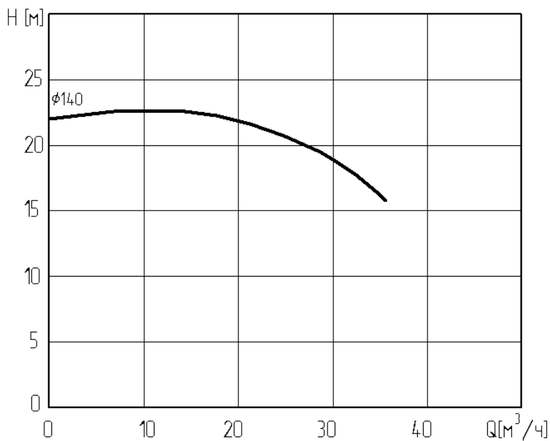
Рис. 1 Рабочие характеристики насоса «Иртыш»: ПД 50/125.140 – 3/2
