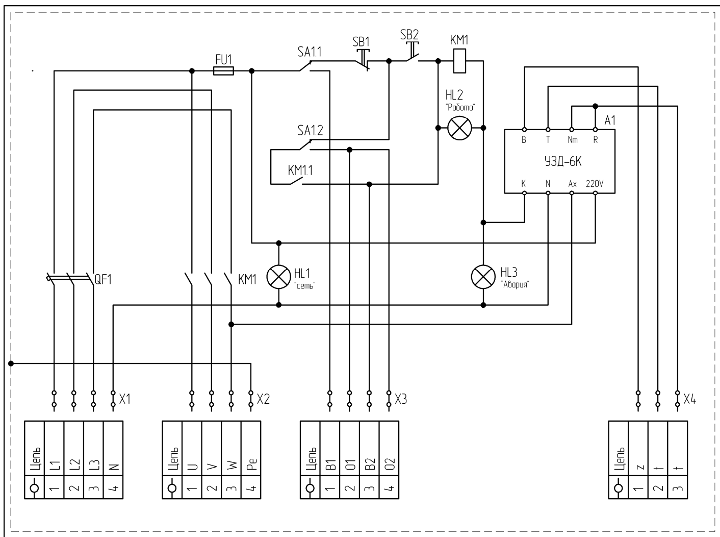
Рис. 34 Принципиальная схема подключения щита управления электронасосов «Иртыш» мощностью от 1,1 до 3кВт.
