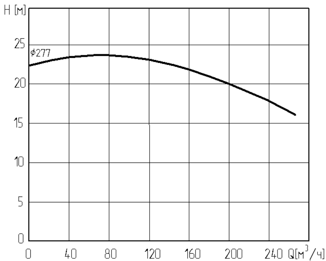
Рис. 5 Рабочие характеристики насоса «Иртыш»: ПД 125/250.277 – 15/4
