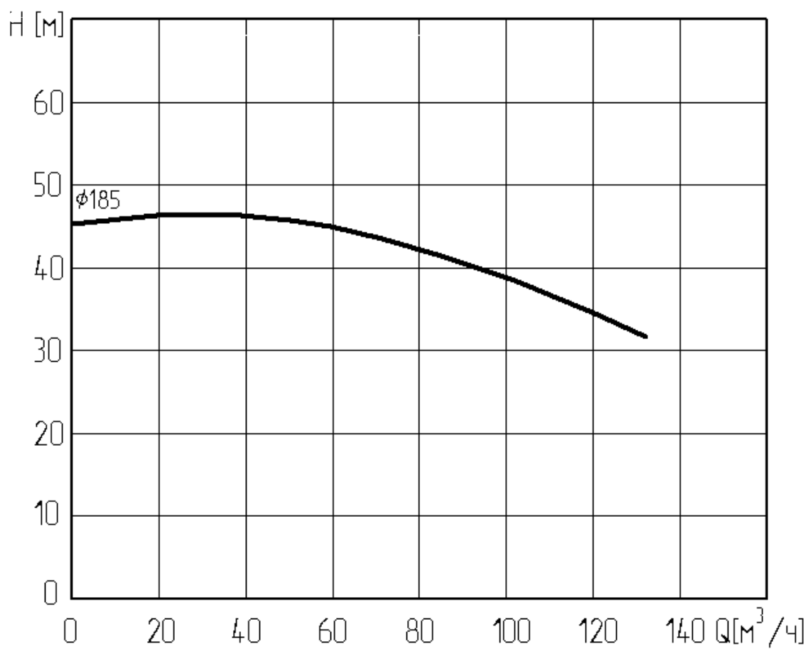
Рис. 3 Рабочие характеристики насоса «Иртыш»: ПД 65/200.185 – 18,5/2
