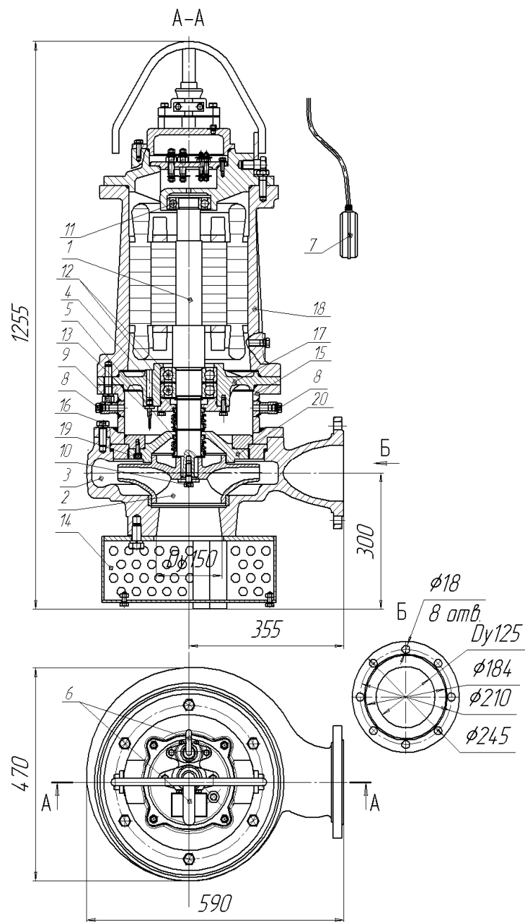
Рис. 16 Общий вид, габаритные и присоединительные размеры электронасоса "Иртыш" ПД 125/315 – 18,5/4
