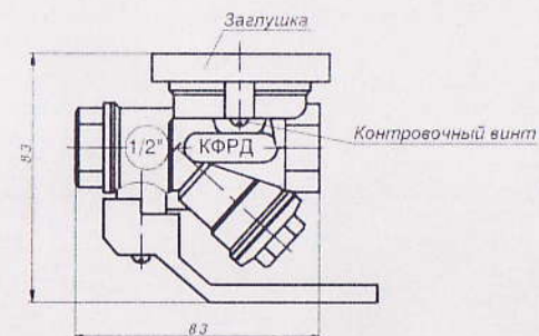
Рисунок 2. Кран-фильтр КФ
