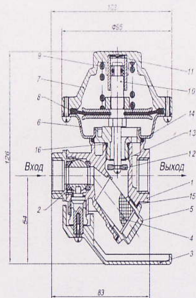
Кран-фильтр
