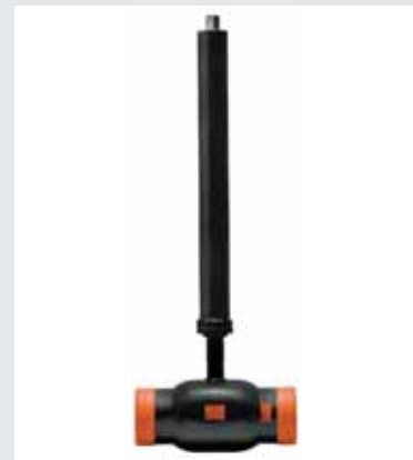
КШТ Серия 21, DN 20-150, PN 2,5/4,0 МПа
