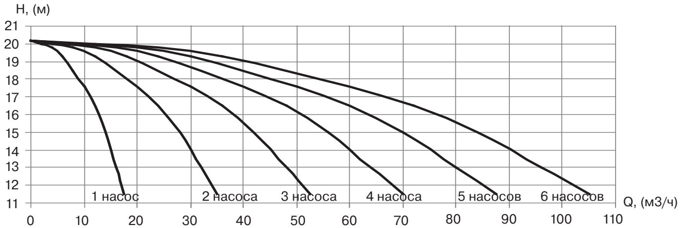
УНВ DPV 25/4 1,1 кВт
