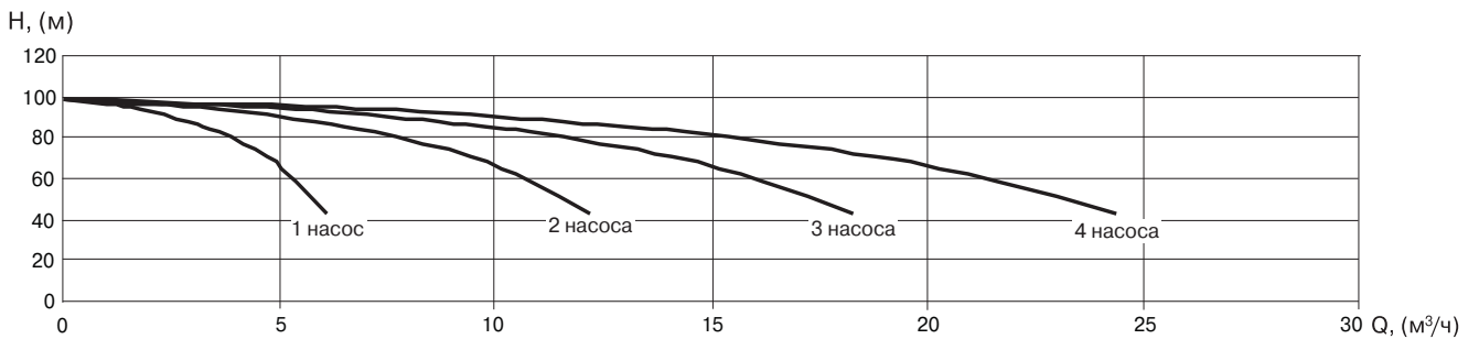
УНВ DPV 4/11
