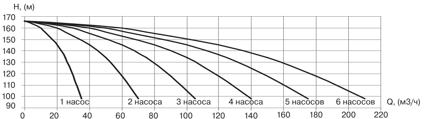
УНВ DPV 25/8 15 кВт
