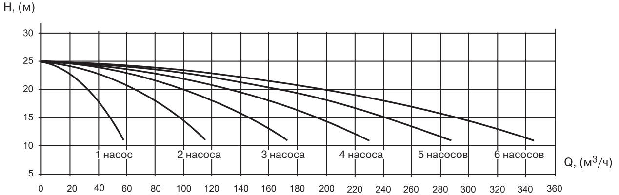
УНВ DPV 45-20-1/5,5
