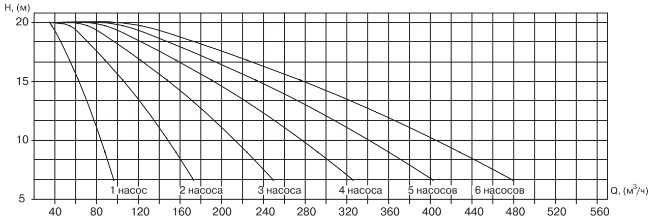
УНВ 3М 65-125/5,5
