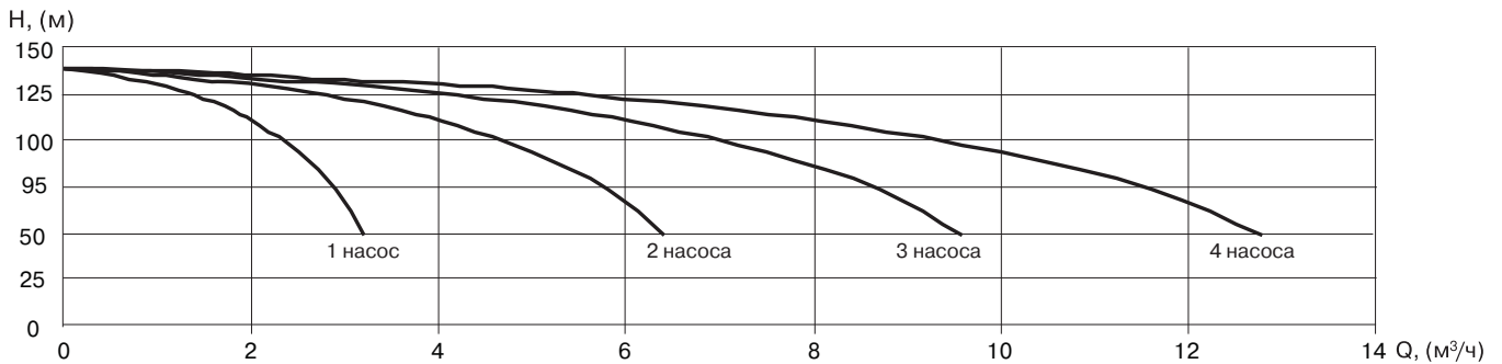
УНВ DPV 2/18
