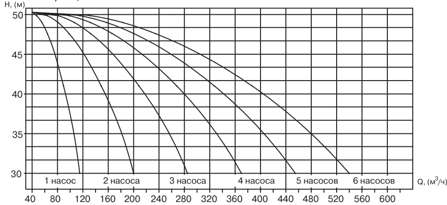
УНВ 3М 65-200/18,5
