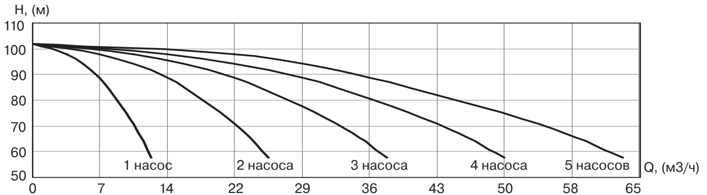
УНВ DPV 10/10 4 кВт
