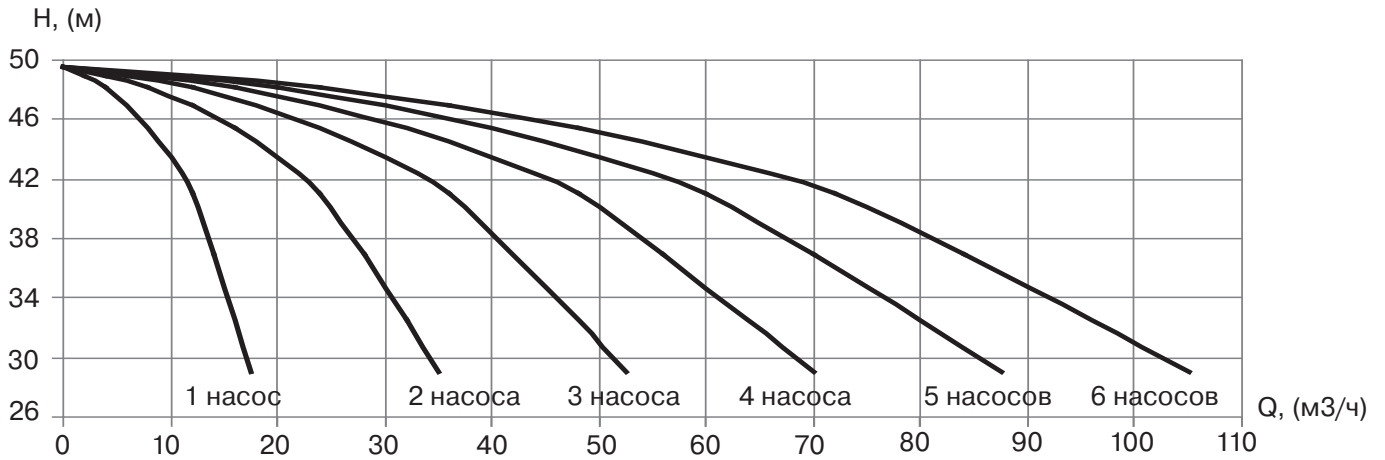
УНВ DPV 25/10 2,2 кВт
