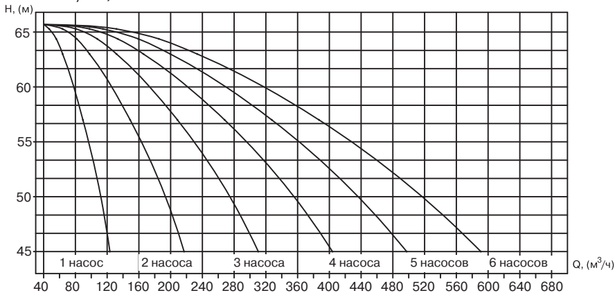
УНВ 3М 65-200/22,0
