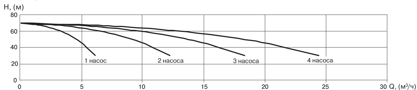
УНВ DPV 4/8
