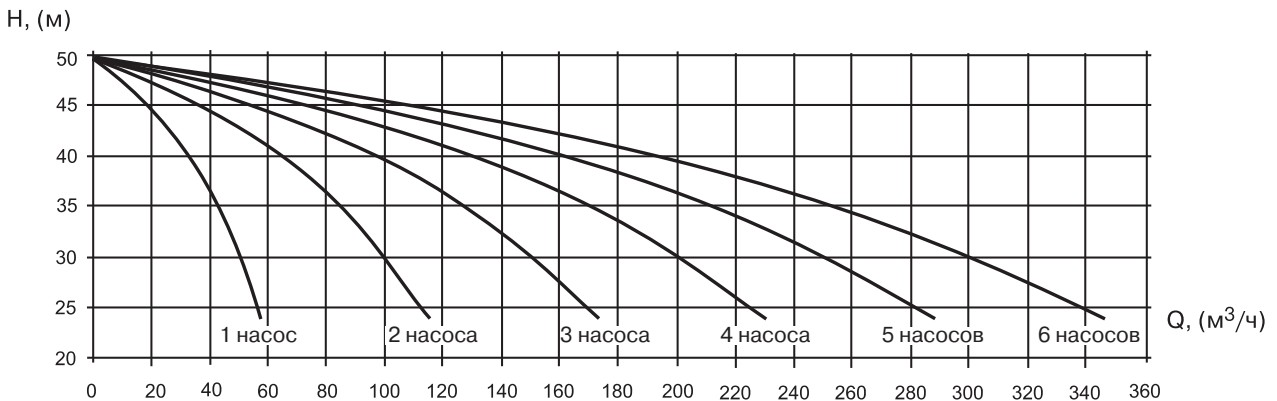
УНВ DPV 45-20/7,5
