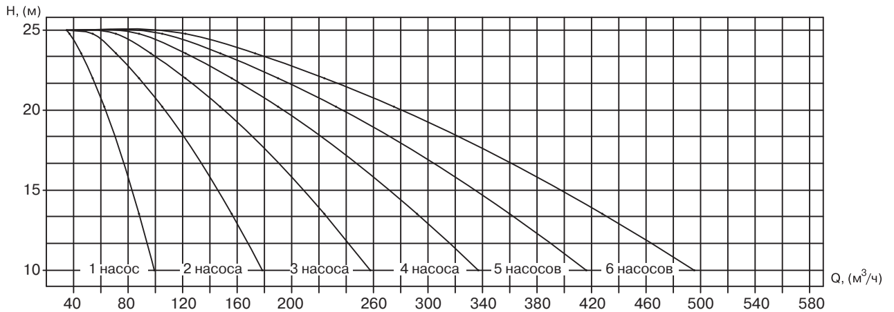
УНВ 3М 65-125/5,5
