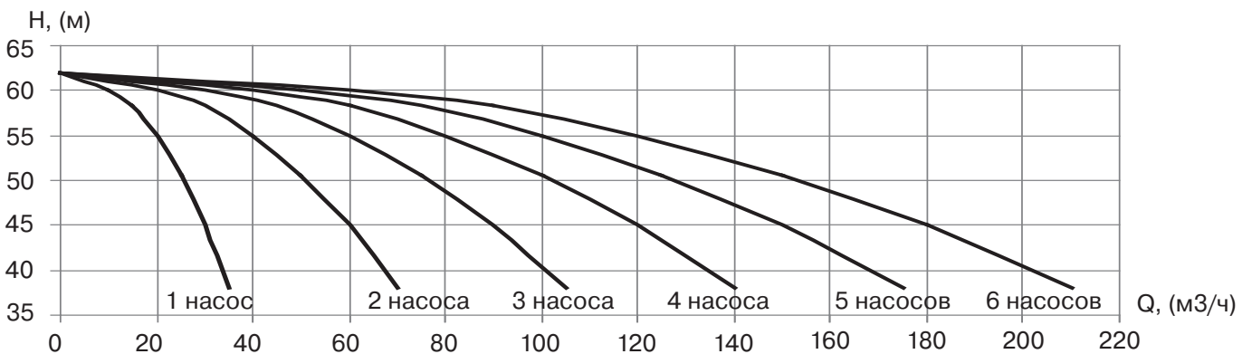
УНВ DPV 25/3 5,5 кВт
