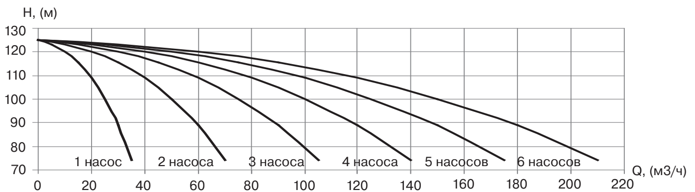
УНВ DPV 25/6 11 кВт
