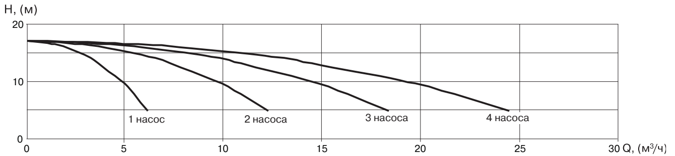
УНВ DPV 4/2
