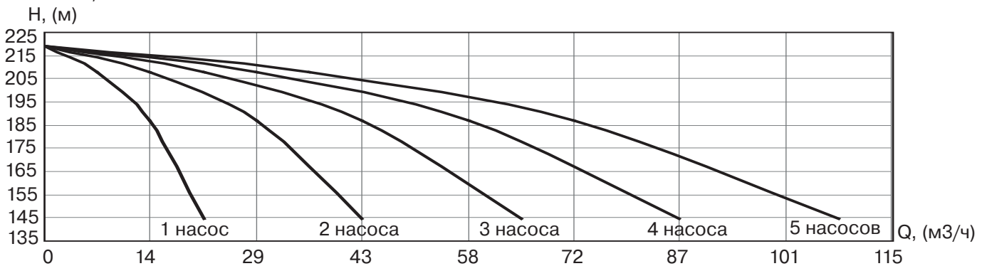
УНВ DPV 15/15 15 кВт
