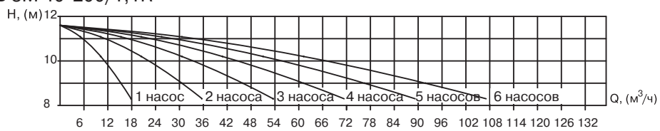
УНВ 3М 40-200/1,1
