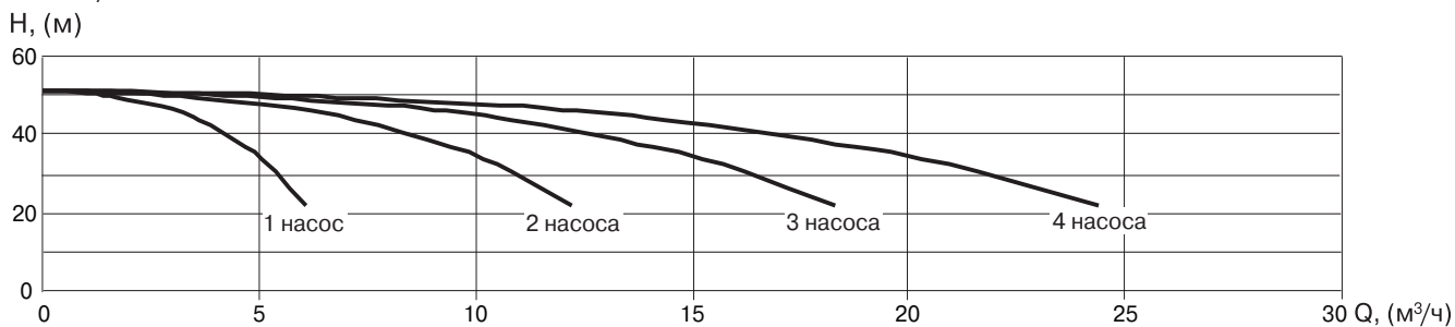
УНВ DPV 4/6
