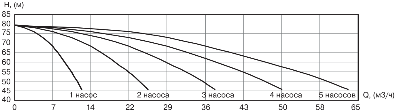
УНВ DPV 10/7 3 кВт
