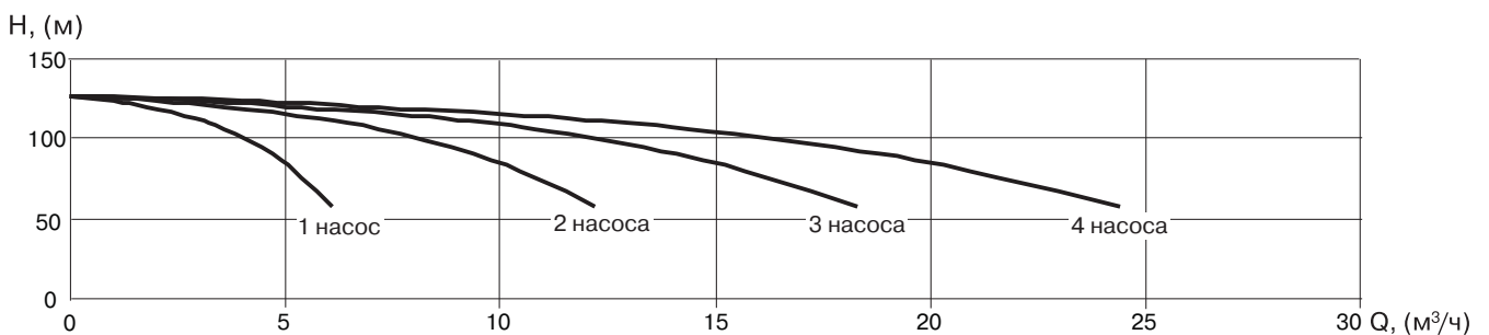
УНВ DPV 4/14
