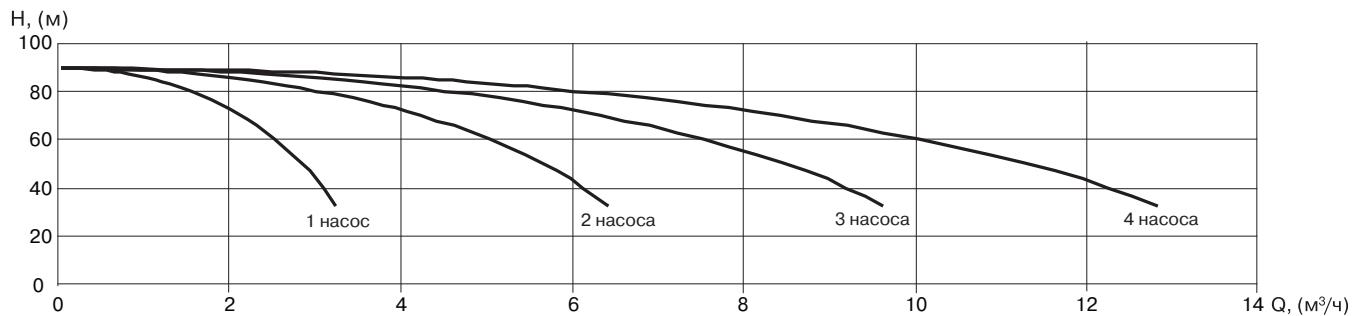
УНВ DPV 2/12
