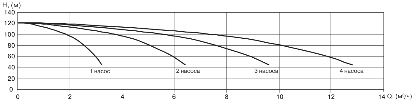
УНВ DPV 2/16
