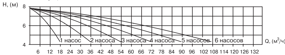
УНВ 3М 40-160/0,55
