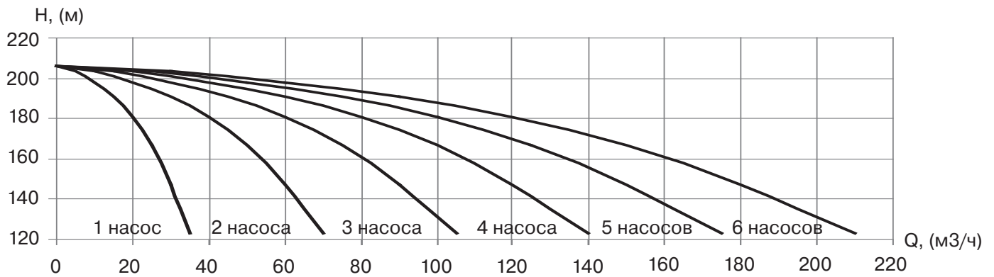
УНВ DPV 25/10 18,5 кВт
