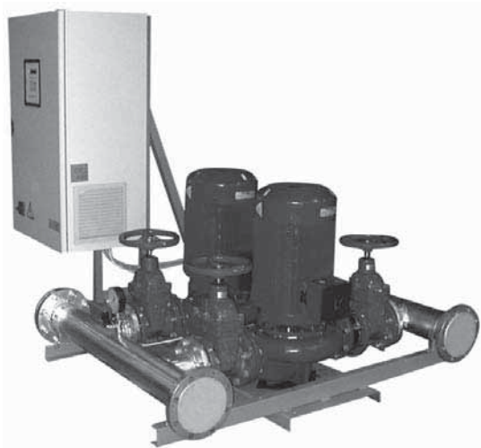
Частотное регулирование с контроллером
