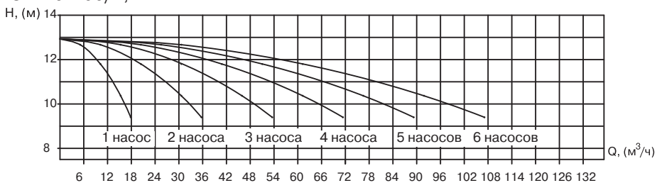
УНВ 3М 40-200/1,5
