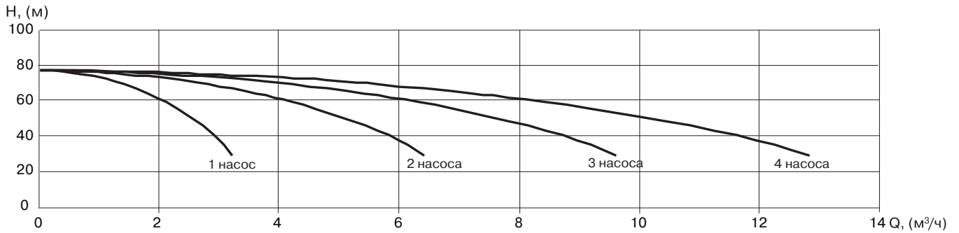
УНВ DPV 2/10
