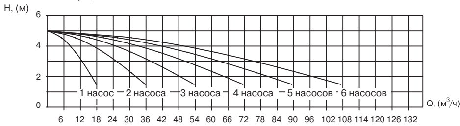
УНВ 3М 40-125/0,37
