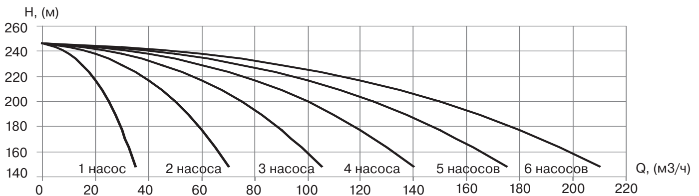
УНВ DPV 25/12 22 кВт
