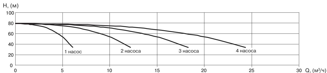
УНВ DPV 4/9
