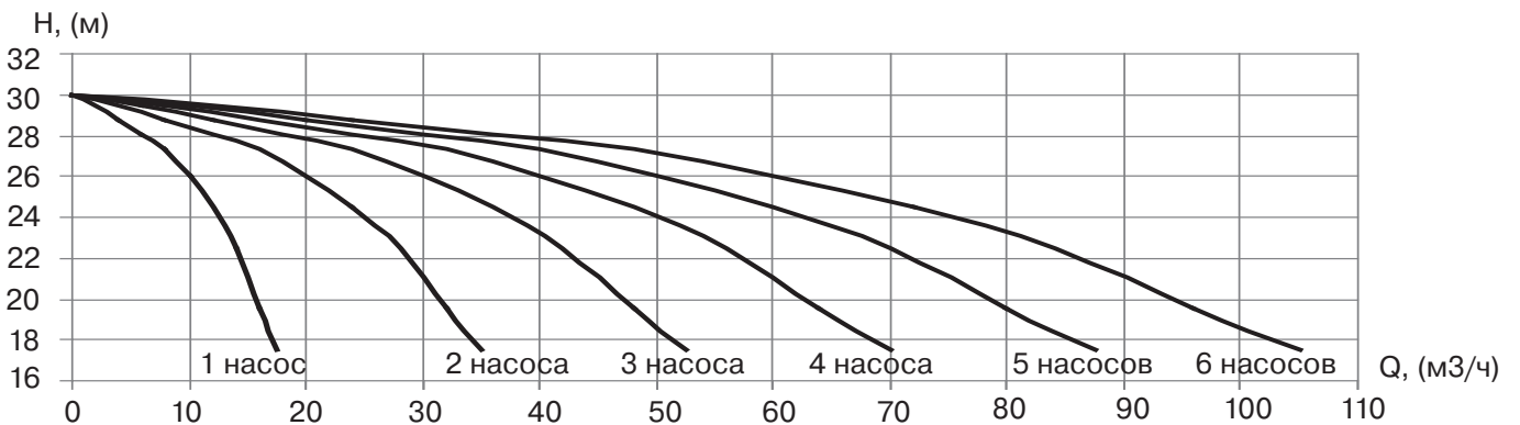
УНВ DPV 25/6 1,5 кВт
