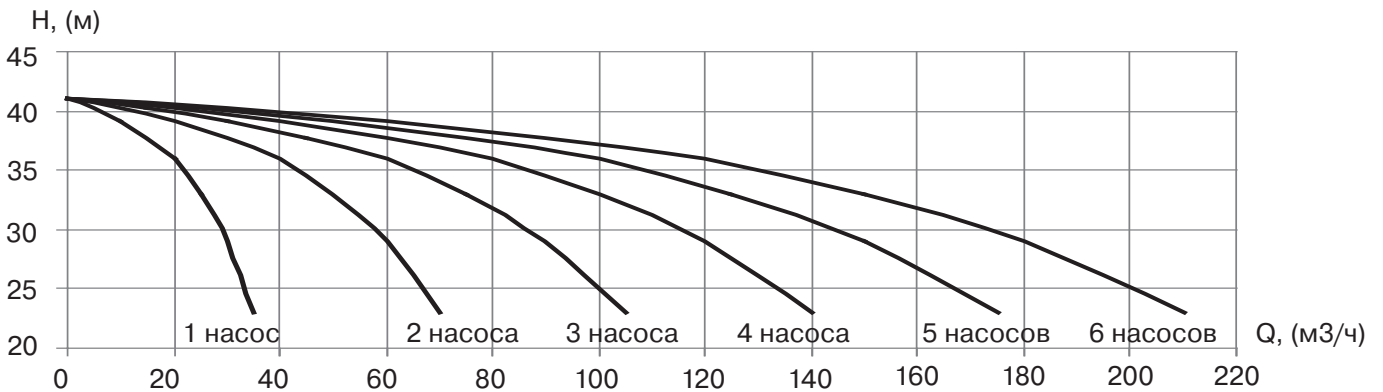
УНВ DPV 25/2 4 кВт
