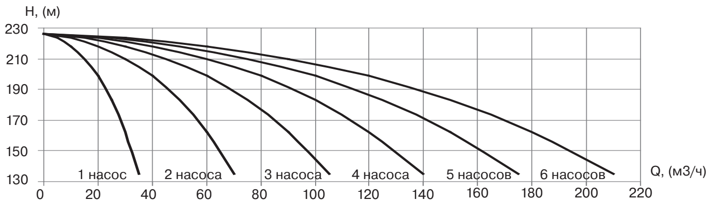
УНВ DPV 25/11 18,5 кВт
