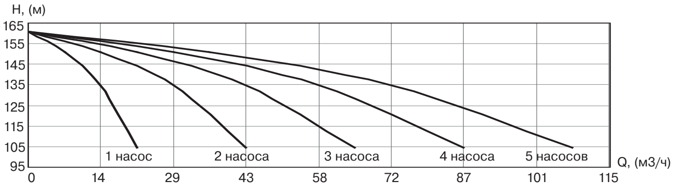
УНВ DPV 15/11 11 кВт
