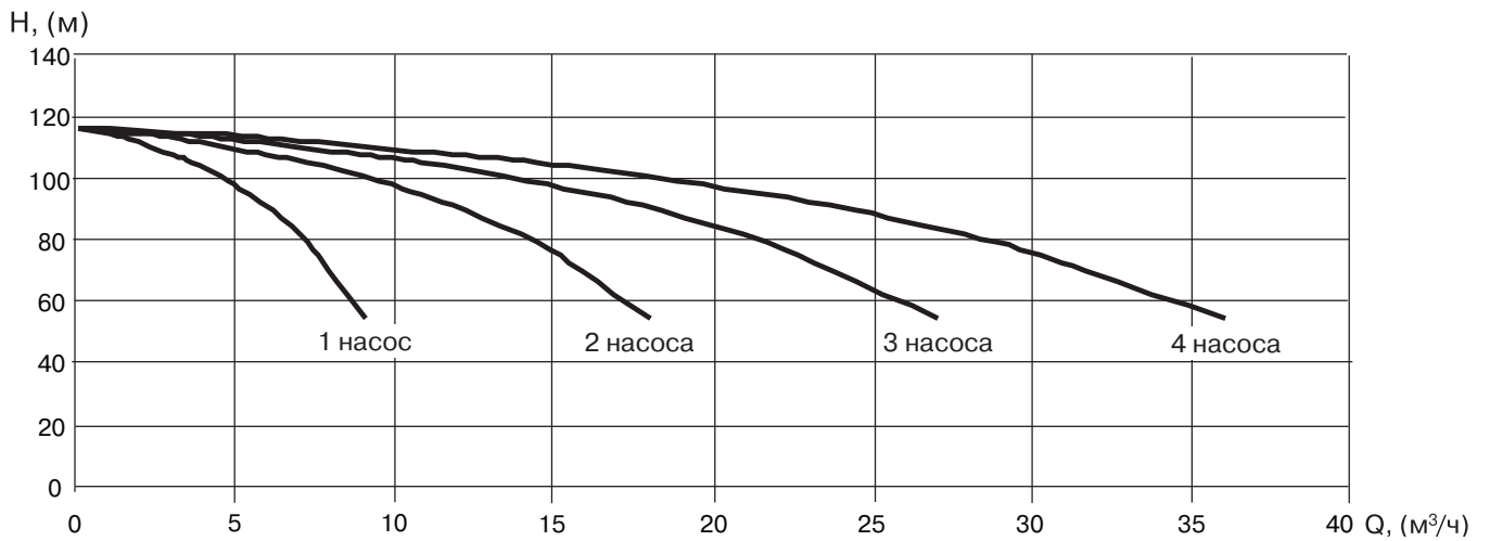
УНВ DPV 6/12
