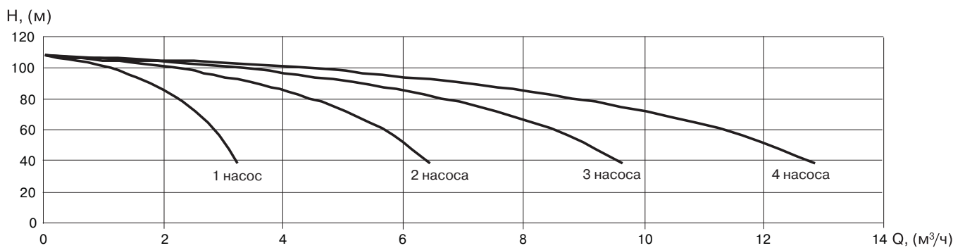
УНВ DPV 2/14
