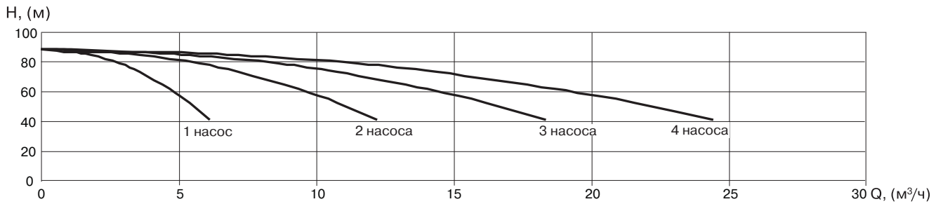
УНВ DPV 4/10
