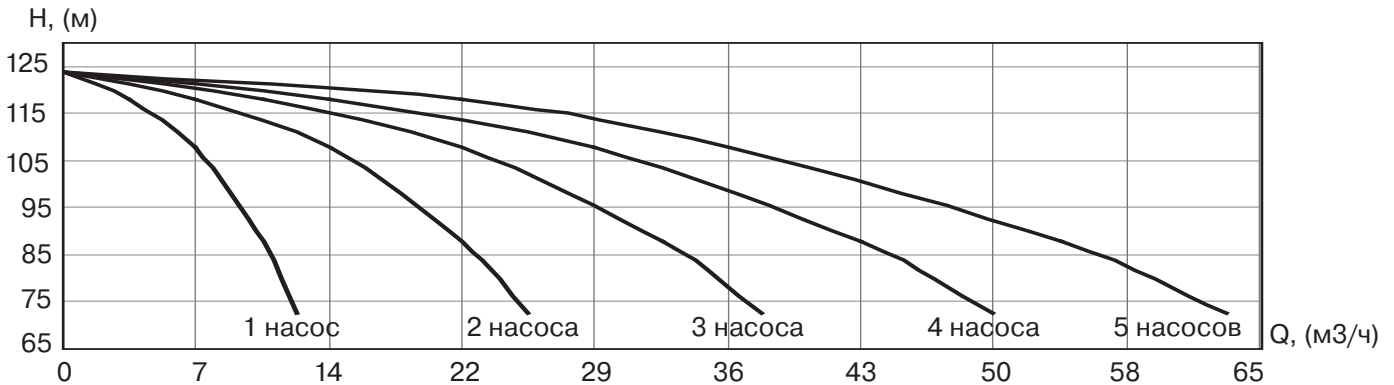
УНВ DPV 10/11 4 кВт
