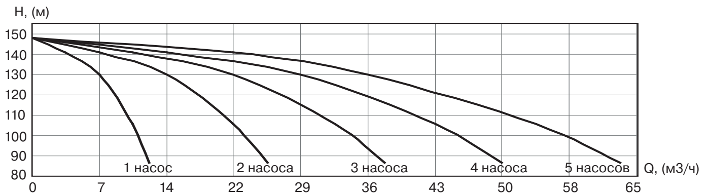
УНВ DPV 10/13 5,5 кВт
