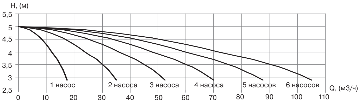
УНВ DPV 25/1 1,1 кВт
