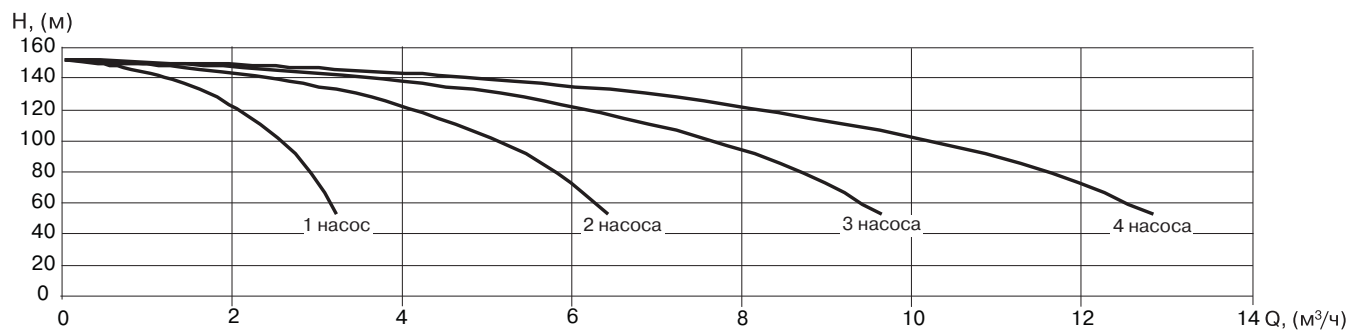
УНВ DPV 2/20
